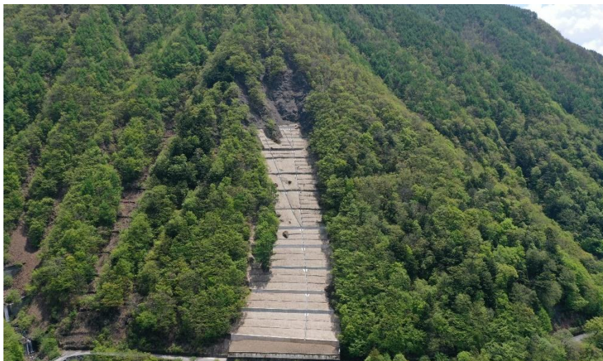
野呂川赤沢崩直轄治山工事 山梨県南アルプス市 清水建設工業（株）
